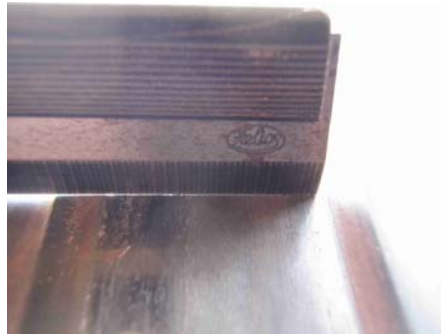
Fuente: P2170195 Superficie de sellado – antigua
