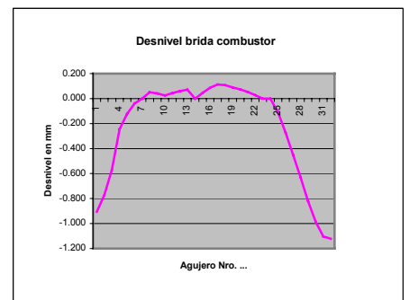
Fuente: 014778.MAQ Reporte de planitud
