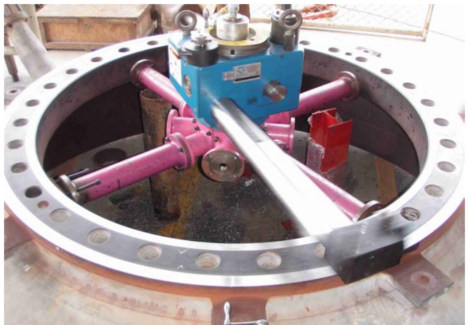
Fuente: P2150160 Refrentadora FF6000, usada para rectificar las superficies de sellado
